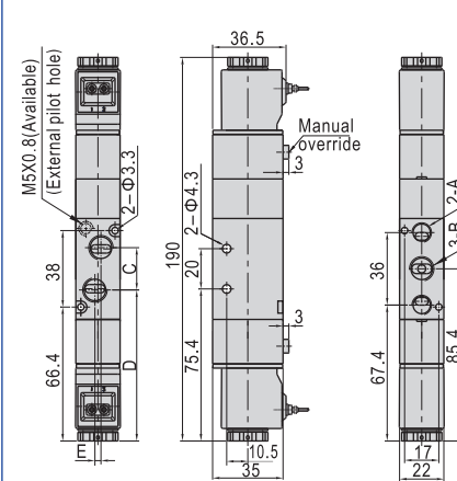
4V230(Grommet)
