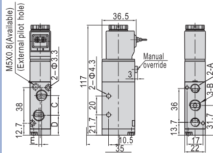
4V210(Grommet)
